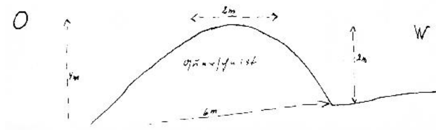
Przekrój wału w Barczewku, MVF, PM-A 060/1, Alt Wartenburg, Kr. Allenstein, wyk. C. Engel.
