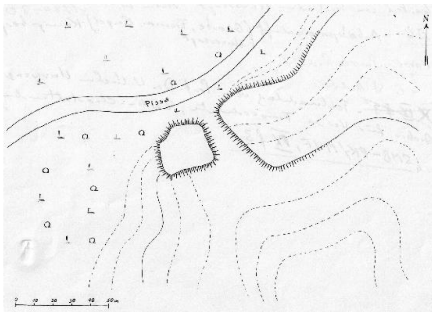
Plan „Krzyżowej Góry” – MVF, IX f3, Burgwallkarte, Wartenburg, Kr. Allenstein, wyk. W. Gaerte.
